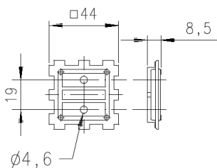
Montážní deska
