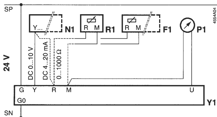
Svorky přípojně svorkovnice
