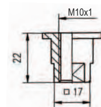
Rozměry spojky
