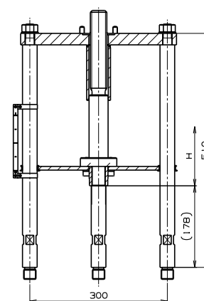
Ovládání DN 600 Připojení A, F10, Tr36x6-LH
