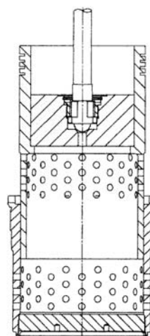
Dvoustupňová redukce tlaku
