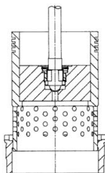
Jednostupňová redukce tlaku
