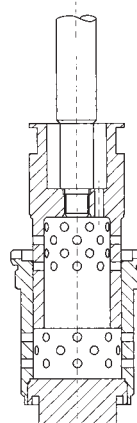
Dvoustupňová redukce tlaku
