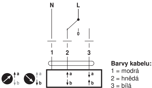
AC 230 V, 3bodové
