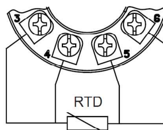
Čtyřvodičové s kompenzací odporu přívodů
