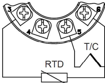
Externí kompenzace st. konce (Pt100 dvovodičově)
