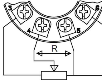
Čtyřvodičové s kompenzací odporu přívodů
