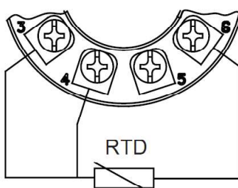
Třívodičové s kompenzací odporu přívodů
