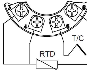
Externí kompenzace st. konce (Pt100 třívodičově)
