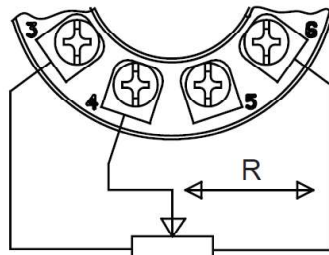
Třívodičové s kompenzací odporu přívodů
