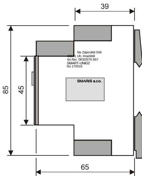
Standardní varianta proudová smyčka 4-20mA
