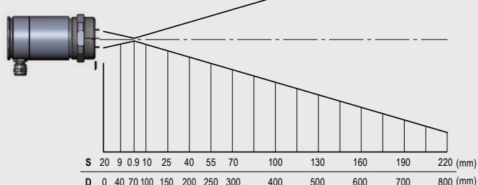
CF3 optics 75:1
