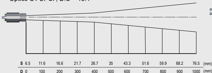
Optics CT LT SF, D:S = 15:1
